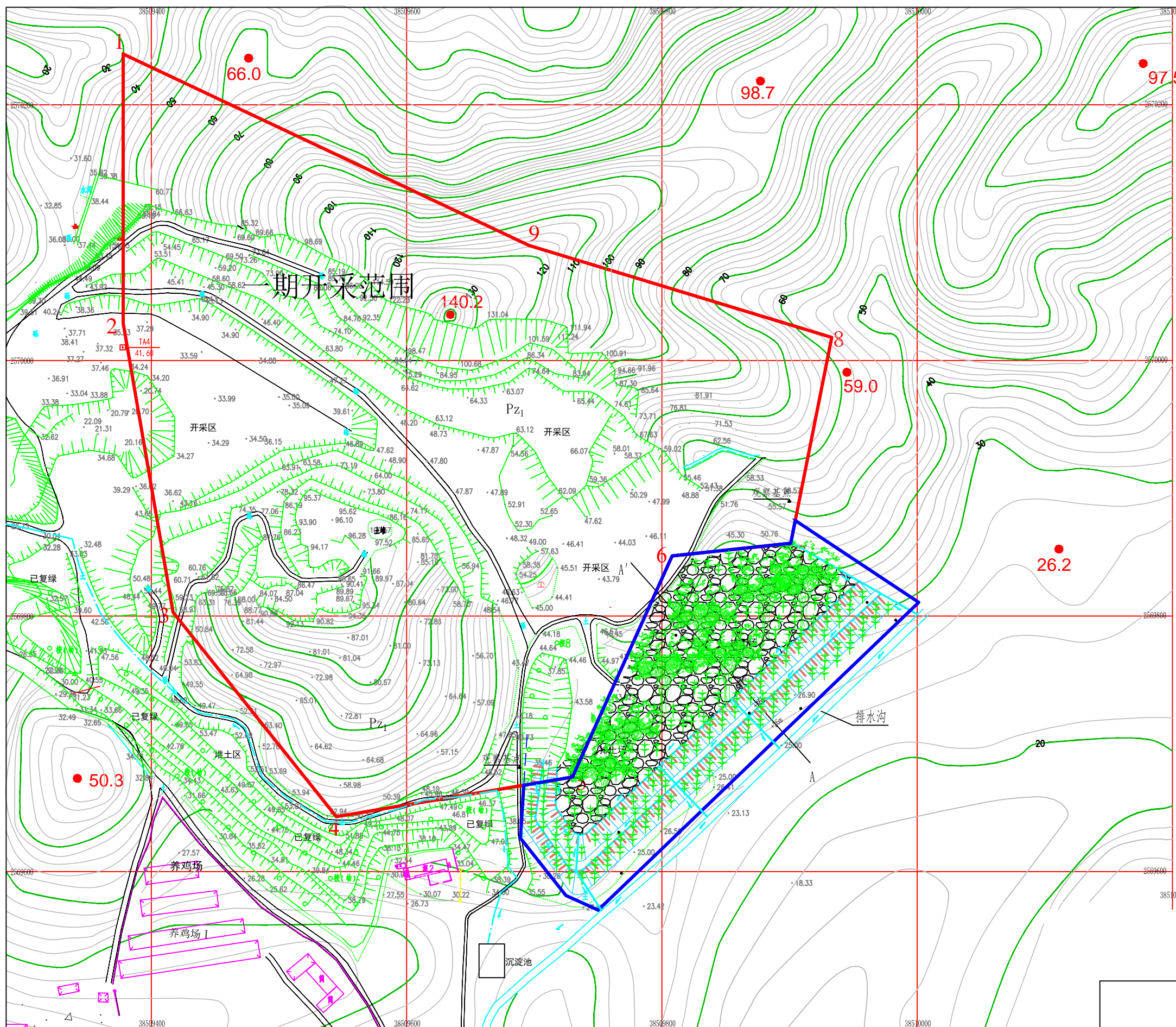
附图4排土场水土保持措施布置平面图
